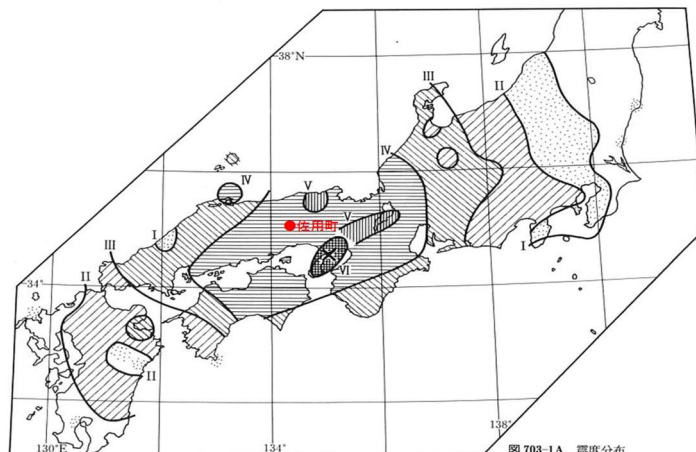
図 703-1A 震度分布
