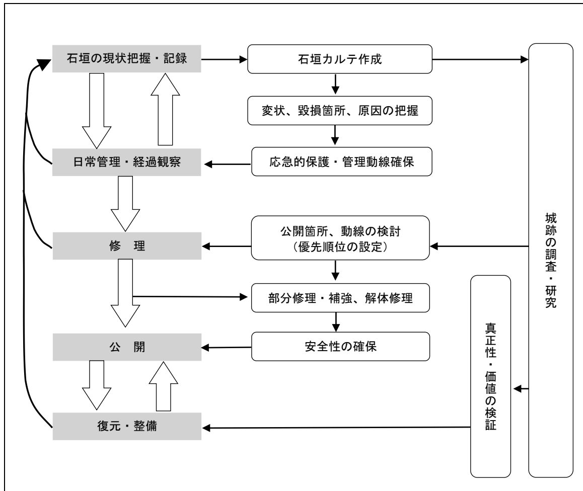
図 8-2 利神城跡石垣の保存管理と整備の関係図
