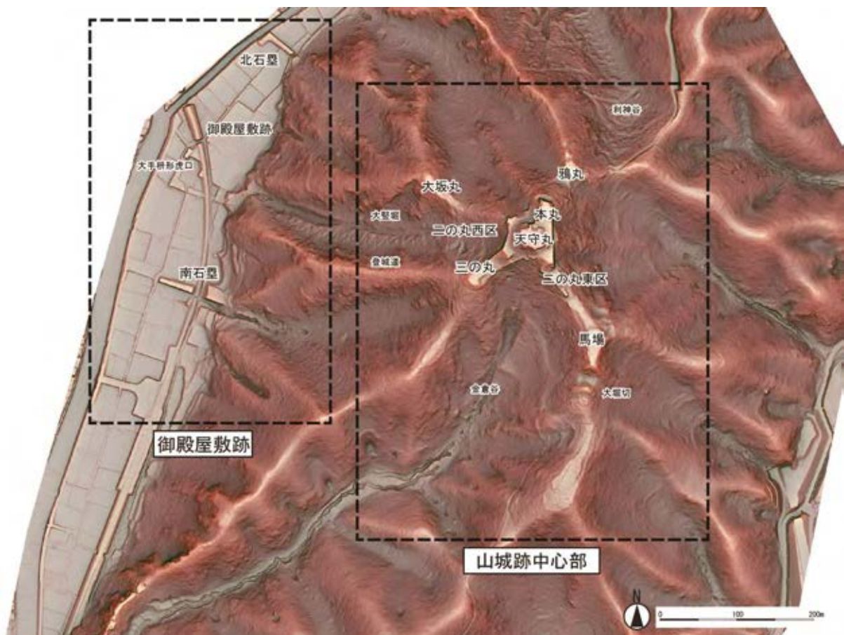
図 3-10 利神城の縄張り ※平成 27 年度（2015）航空レーザー計測による赤色立体図
