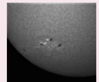
H \alpha 線太陽望遠鏡がとらえた太陽フレアの瞬間 (白く光っている部分がフレア)
