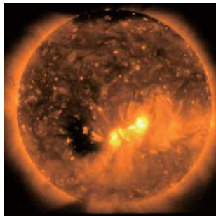
太陽観測衛星「ひので」が撮影した黒い太陽とその周囲のコロナ
