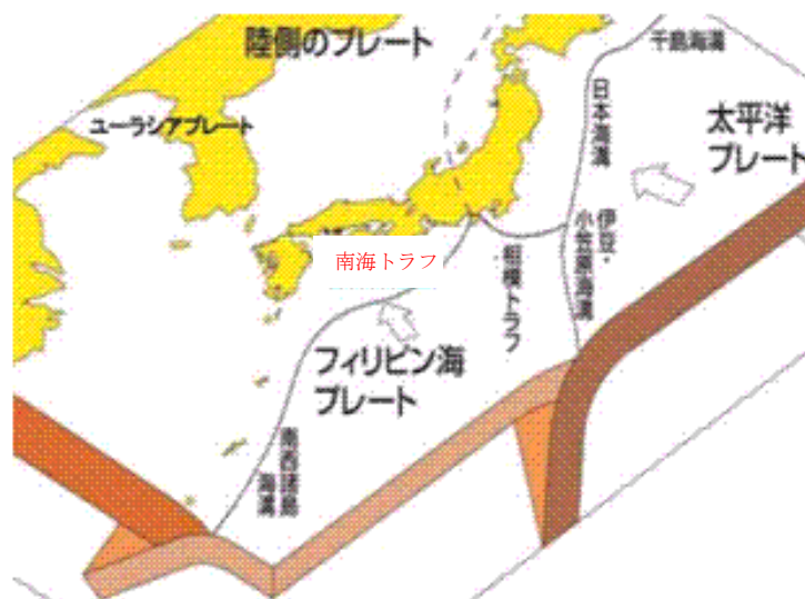
図：日本近辺のプレート
